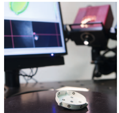
Optische Analyse der Bauteilgeometrie eines tiefgezogenen Bauteils mit integrierten Nebenformelementen
